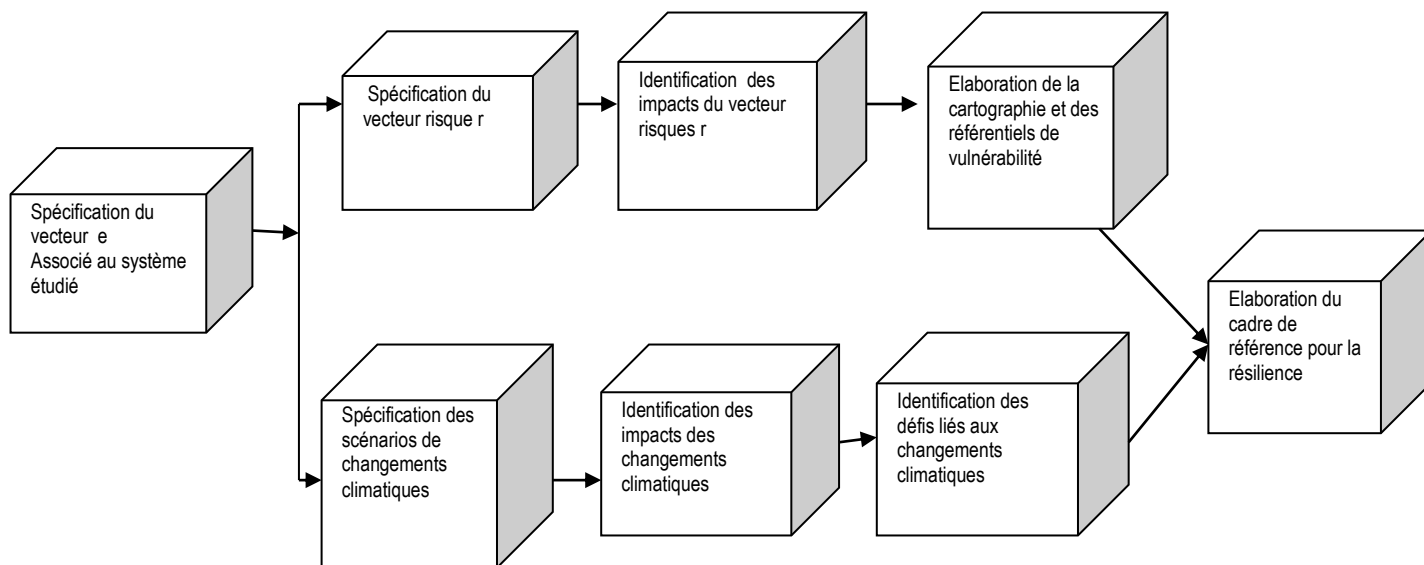
Figure (3) : illustration schématique du modèle ClimProspect
